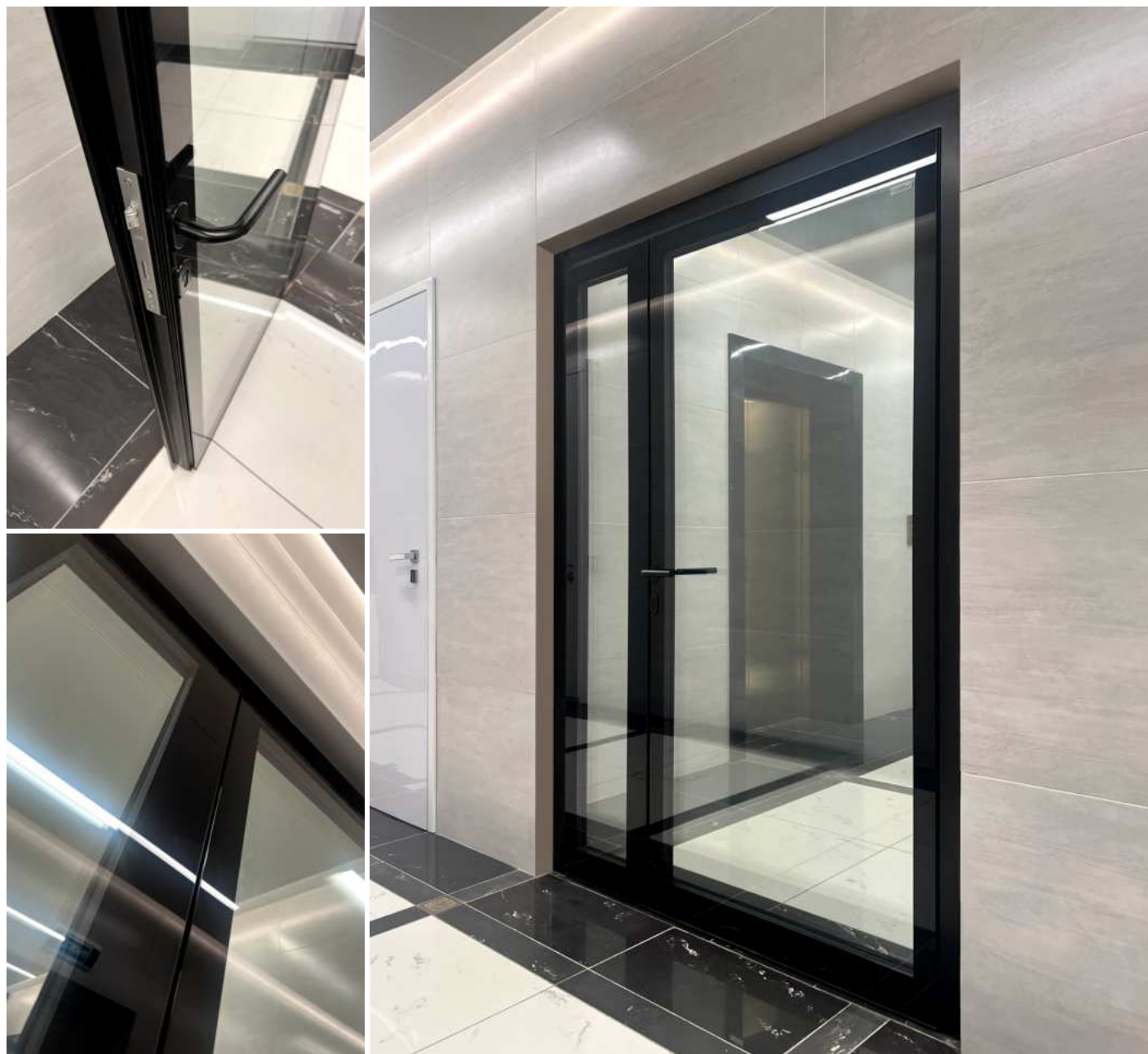
Фото готовой продукции – противопожарная дверь EIWS-60 – стеклопакет и полотно в единой плоскости. Установлена в лифтовом холле столичного ЖК
